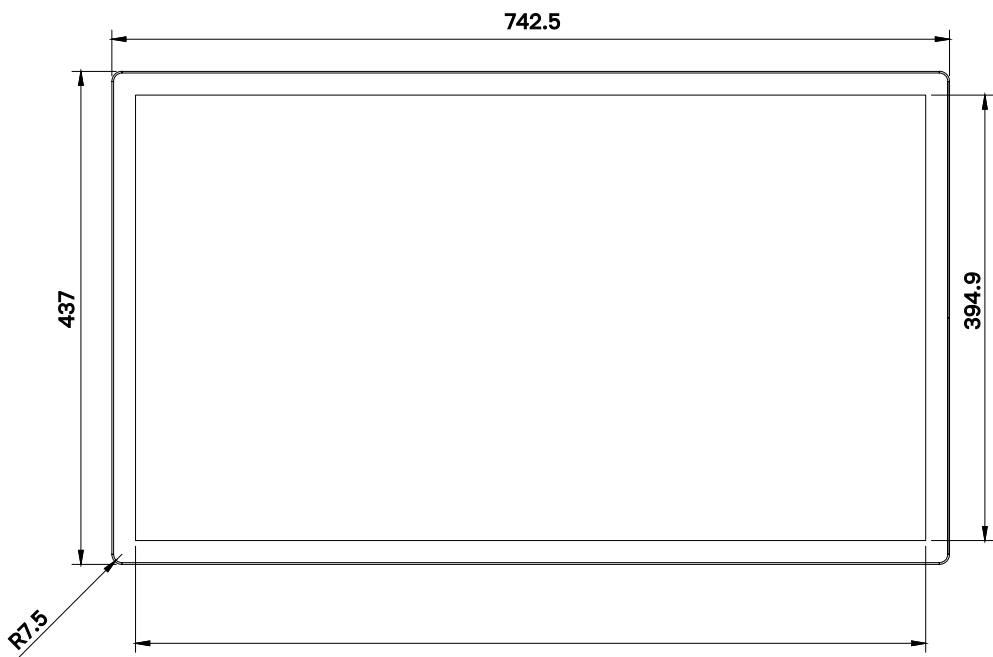
СХЕМА ДИСПЛЕЯ (ВИД СПЕРЕДИ)
