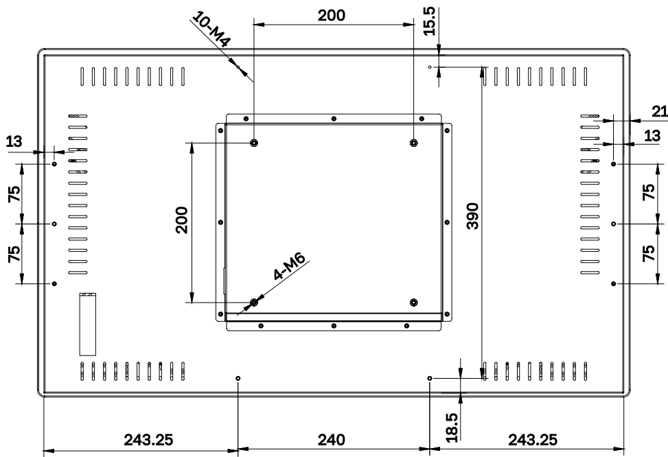
СХЕМА ДИСПЛЕЯ (ВИД СЗАДИ)
