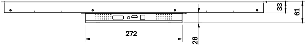
СХЕМА ДИСПЛЕЯ (ВИД СВЕРХУ)
